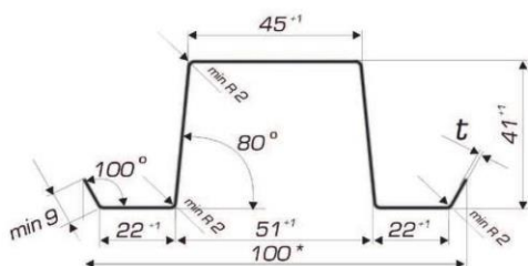
Обрешеточный профиль
