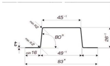
Стеновой профиль
